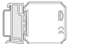
c) Ad aggancio avvenuto, collegare la linea bus, gli ingressi e le uscite
